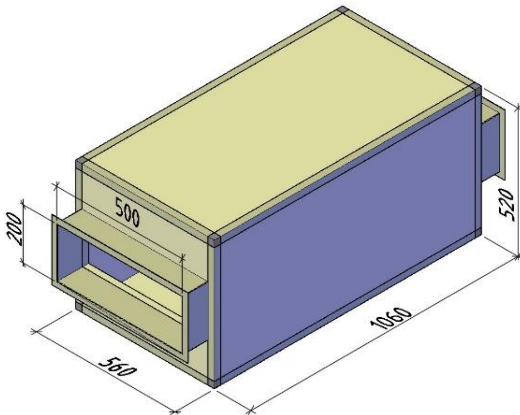
AVI E 13.5/380/2000 Размеры: 1060x560x520мм 500x200мм
